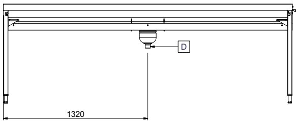
Zij aanzicht
